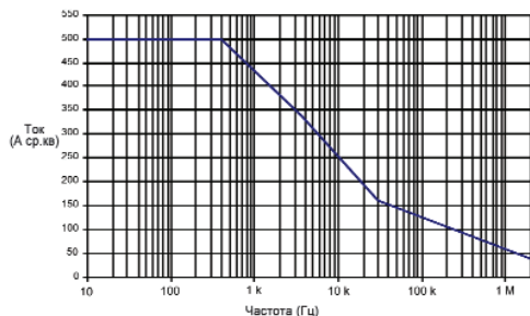
Максимальный входной ток при частоте
