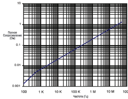
Полное вносимое сопротивление при частоте
