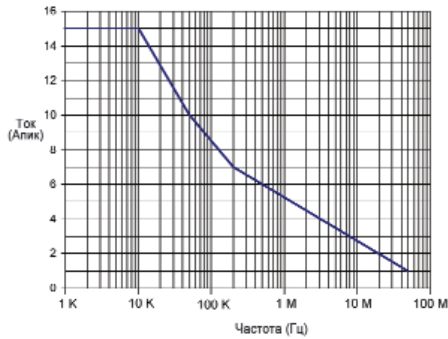
Максимальный входной ток при частоте
