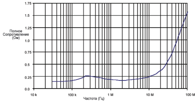
Полное сопротивление пробника в зависимости от частоты
