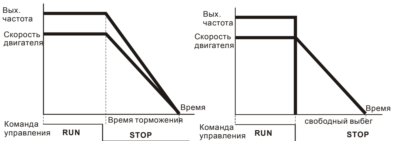
Остановка с замедлением и на выбеге
