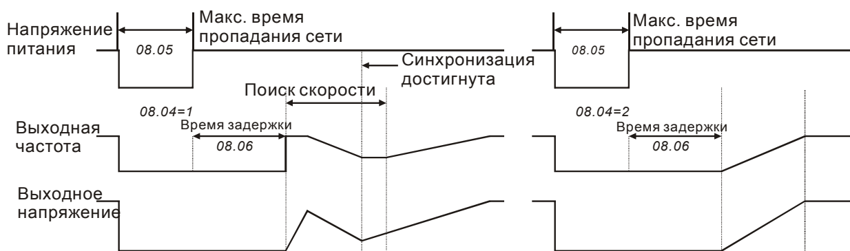
Рестарт после пропадания напряжения питания
