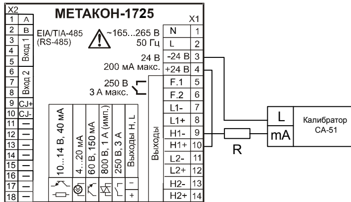
Рисунок А.9 – Схема подключения прибора для проверки основной погрешности установления тока в токовом выходе, где R – резистор C2-33H-0,125-200 Ом ± 5 %.
