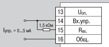
Ток 0...5 мА
