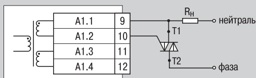
Симистор
