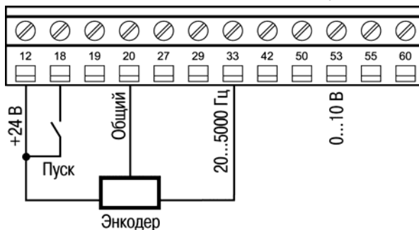
Рисунок 3.15 – Схема подключения энкодера с питанием от встроенного источника питания ПЧВ
