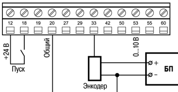
Рисунок 3.16 – Схема подключения энкодера с питанием от внешнего источника питания
