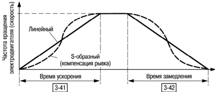
Рисунок 3.1 – Характеристики разгона/торможения
