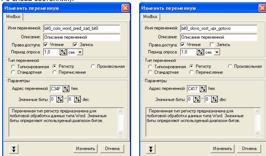
Рисунок 4.19 - Настройки для отображения 0-х битов командного слова и слова состояния
