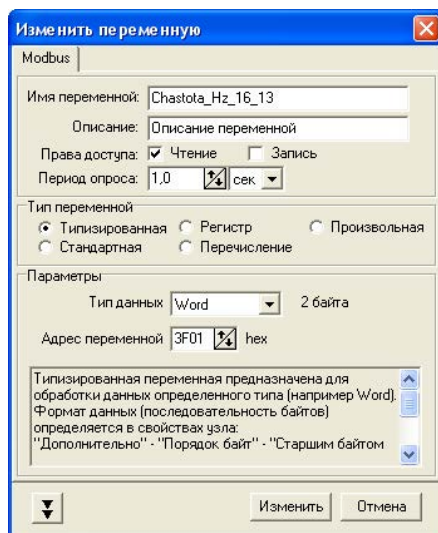
Рисунок 4.15 - Настройка переменной ПЧВ 16-13 Частота, Гц для отображения в OPC
