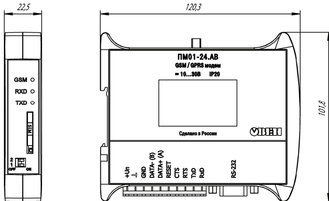
Рисунок А.1 – Габаритный чертёж модема
