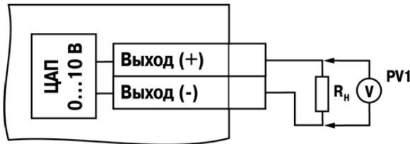
Рисунок Б.7 – Схема подключения нагрузки к ВЭ типа «У». R_H > 2 \text{ кОм}
