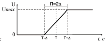
б) прямо-пропорциональное регулирование
