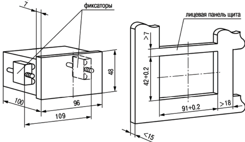
Рисунок А.2 – Прибор щитового крепления Щ2
