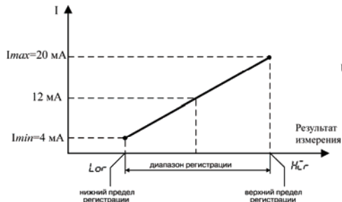
Рисунок 3.7 – Принцип формирования выходного сигнала ВУ в режиме регистратора для приборов с ВУ типа И
