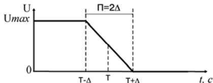
а) обратно-пропорциональное регулирование
