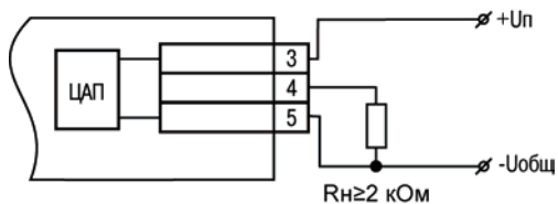
Рисунок Б.8 – Пример подключения ВУ типа У
