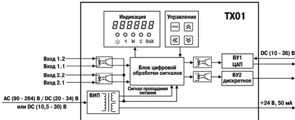
Рисунок 3.1 – Функциональная схема
