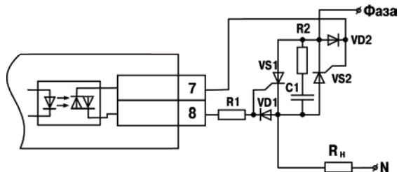
Рисунок Б.5 – Схема подключения силового симистора к ВУ типа С
