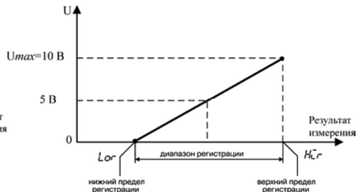
Рисунок 3.8 – Принцип формирования выходного сигнала ВУ в режиме регистратора для приборов с ВУ типа А
