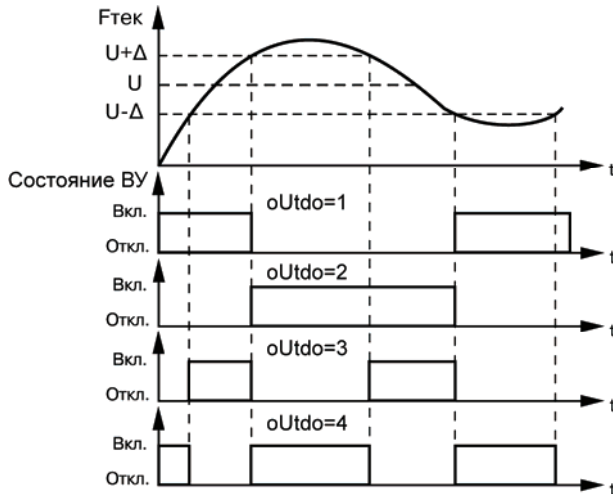
Рисунок 3.4 – Типы логики при работе ВУ в качестве компаратора
