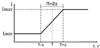
б) прямое пропорциональное регулирование
