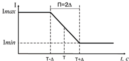
а) обратное пропорциональное регулирование
