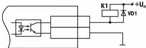
Рисунок 3.6 – Использование транзисторной оптопары для управления реле
