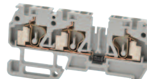
DN-Q12-1-2DR-A (Euro QM2.5/35)
