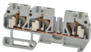
DN-Q12-1-2-A (Euro QM2.5/35)
